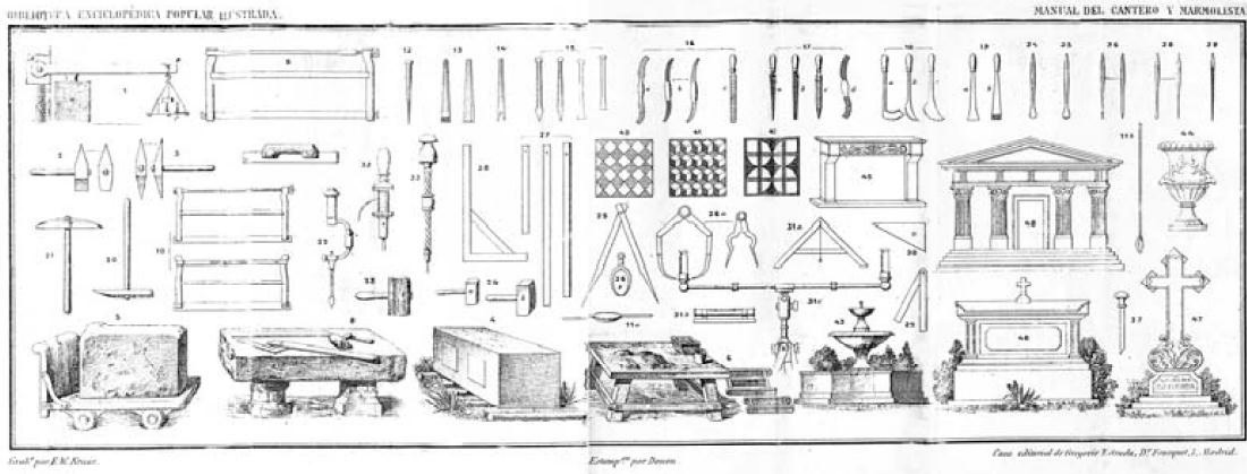
Figura 1: Antonio Sánchez Pérez, Manual del cantero y del marmolista (Madrid, 1884). (Nota: solo se identifican las figuras relacionadas con el texto) 2.martillo 3.pico 4.bloque arrastrado por rodillos 5.carretón 8.banco 9.sierra 10.serrucho 11.cucharón 12.puntero 13.gradina 14.dos dientes 15.cinceles 16.escofinas 17.limas 18.rodela 19.rascadores 20.martillo 21.pico 22.berbiquí 23.mazo 24.macetas 25.compases 26.compás de gruesos 27.reglas 28.escuadra 29.falsa escuadra 30.plantilla 32.violín 33.espiral 34.mediacaña gradina 36.calados 37.buril 38.brocas 39.limatón
